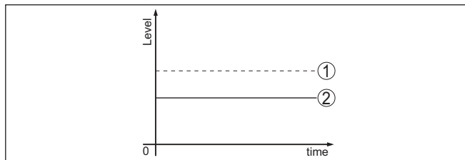
Рис. 18: Пунктирная линия 1 показывает действительный уровень, сплошная линия 2 показывает выдаваемый датчиком уровень
