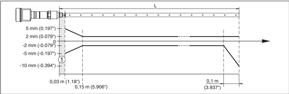
Рис. 20: Погрешность измерения NivoGuide 8200 в коаксиальном исполнении, измерительная длина до 1,5 м/4.92 ft (среда - вода)
