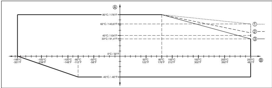
Рис. 24: Температура окружающей среды - температура процесса, стандартное исполнение
