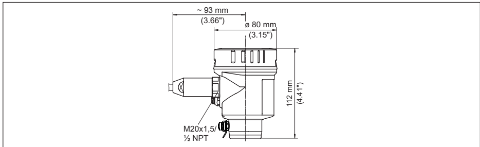
Рис. 28: Корпуса в исполнении IP 66/IP 68 (1 bar), (с установленным модулем индикации и настройки корпус выше на 9 мм/0.35 in)
