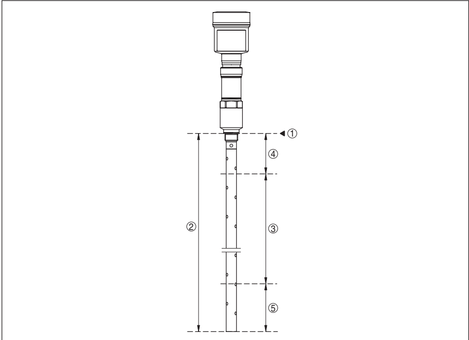
Рис. 19: Диапазоны измерения - NivoGuide 8200
