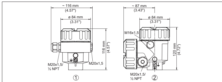
Рис. 25: Корпуса в исполнении IP 66/IP 68 (0,2 bar), (с установленным модулем индикации и настройки корпус выше на 9 мм/0.35 in)
