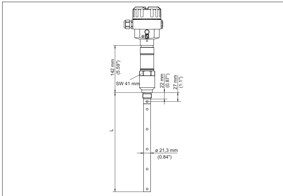
Рис. 29: NivoGuide 8200, коаксиальное исполнение с резьбовым присоединением (-20 ... +250 °C/-4 ... +482 °F)
