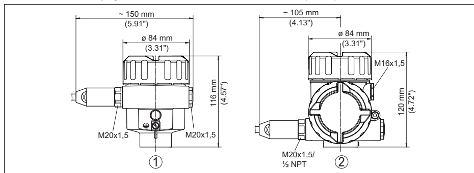
Рис. 26: Корпуса в исполнении IP 66/IP 68 (1 bar), (с установленным модулем индикации и настройки корпус выше на 9 мм/0.35 in)
