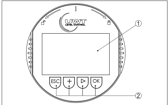
Рис. 16: Элементы индикации и настройки
