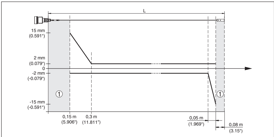
Рис. 34: Погрешность измерения NivoGuide 8100 в тросовом исполнении \varnothing 2 mm/0.079 in (среда - масло)
